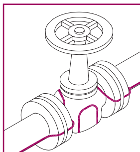
Пример использования кабеля для обогрева трубопровода
